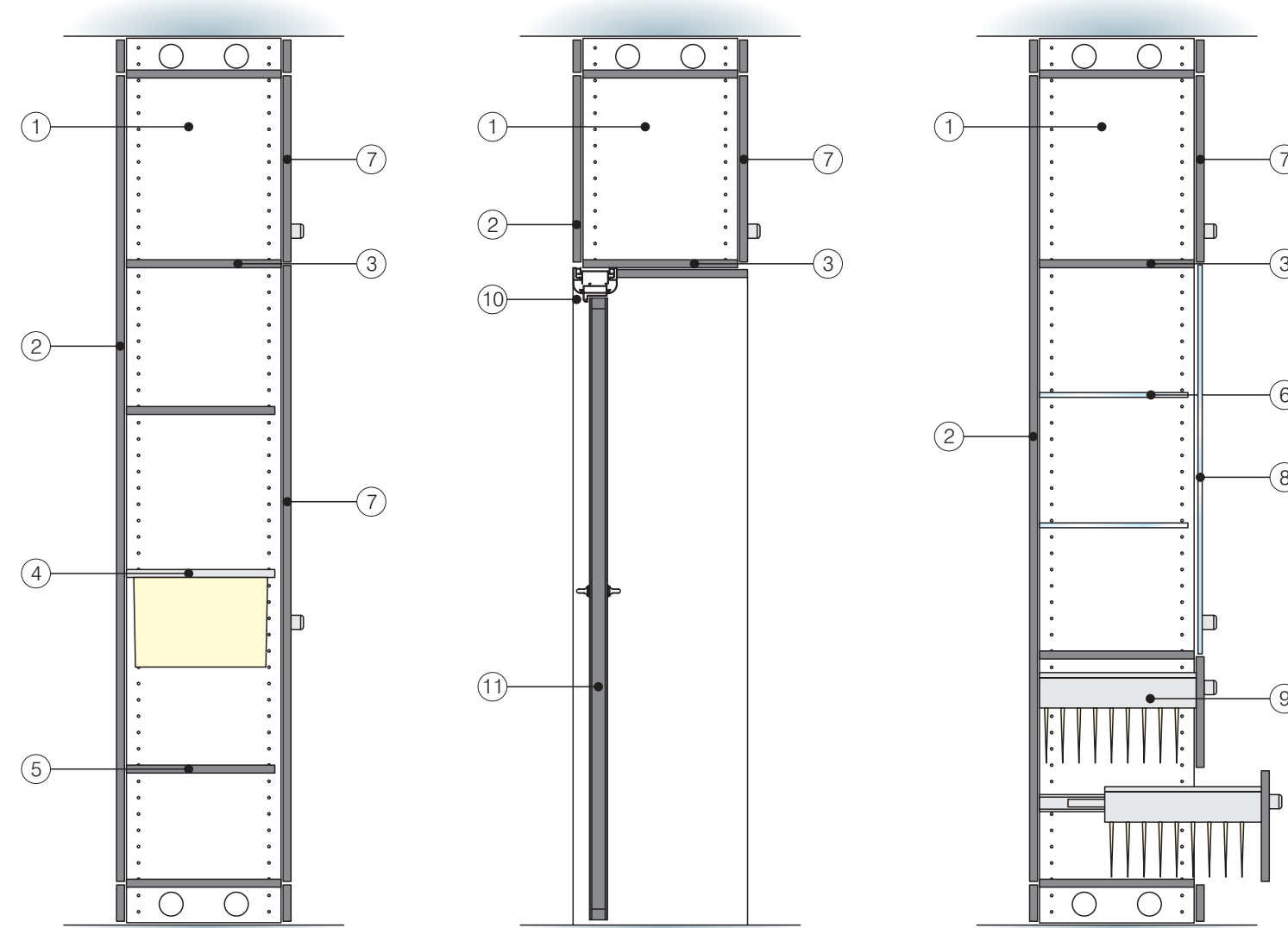
Mobile con ante in legno Unit with wood door
