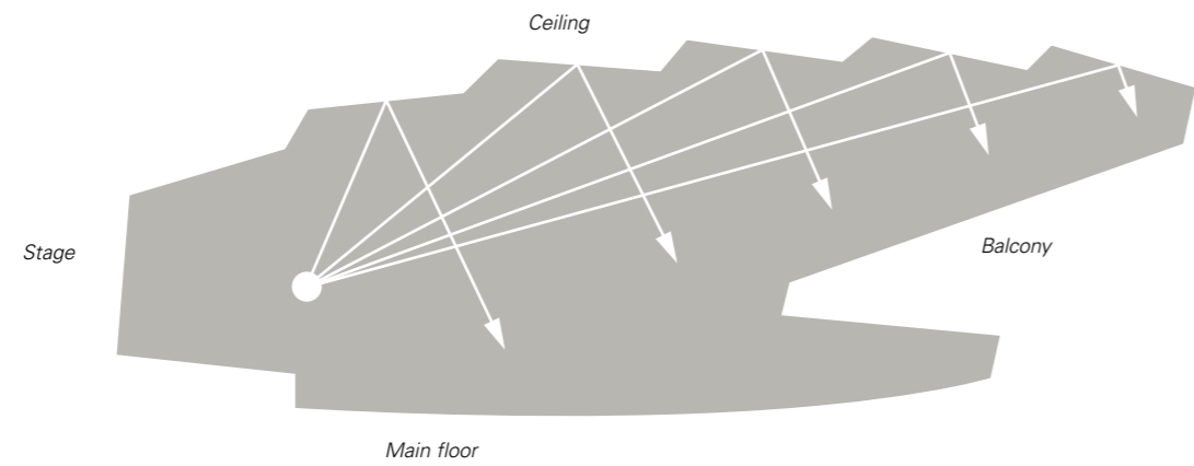
Ricostruzione grafica delle riflessioni delle onde sonore in una sala concerti. Graphical reconstruction of sound waves reflecting inside a concert hall. Grafische Rekonstruktion der Schallreflexion in einem Konzertsaal. Reconstruction graphique des réflexions des ondes sonores dans une salle de concert. Reconstrucción gráfica de las ondas sonoras en una sala de conciertos.
